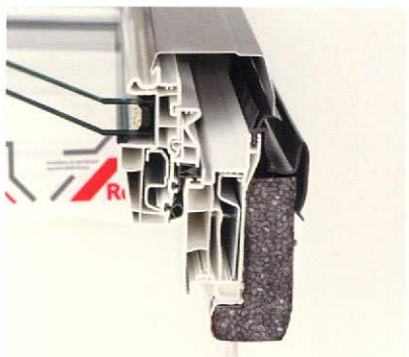
Roto R4/R7 típusú műanyag tetőtéri ablak gyárilag előszerelt Hőszigetelő Csomaggal és belső fóliacsatlakozással.
